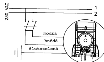
elektrické zapojení
